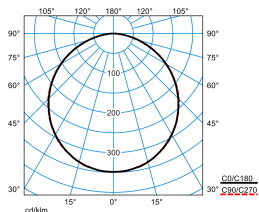
Olisq QWD3 DW 30-830 ETBLE +DMR IP54 IK + Olisq QWD3 ZDR 1/1 03
