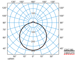
Olisq QWD3 DW 30-830 ETBLE +DMR IP54 IK
