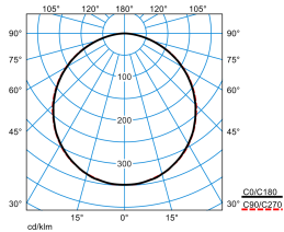
Olisq QWD3 DW 30-830 ETBLE +DMR IP54 IK + Olisq QWD3 ZDR 1/1 01
