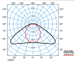
Nextrema G3 XB 6000-840 ET +LV PC TX770686
