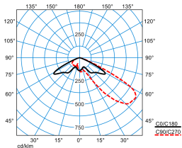
LnPlus 60-AM19L-LR/20000-740 16G1 ET (CLO end value)
