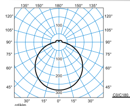
Olisq RWD2 DW 20-840 ETBLE +CAS-S IP54
