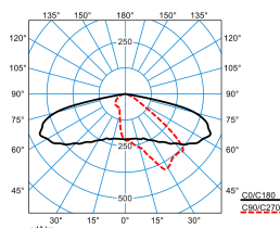
LIQ 50N-AB2L-LR/2000-730 2G1 ET (CLO end value)
