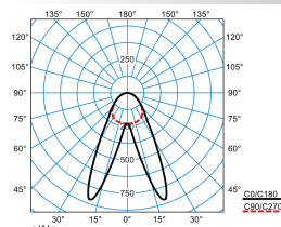
Cflex H1-E DA 3500-840 ET EB3 I2
