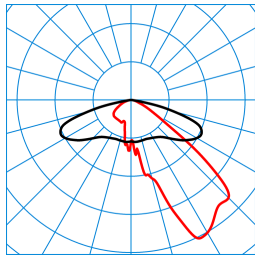
Publisca P2-AB2L/3500-740 4G1S TX047721 ■ C0 - C180 ■ C90 - C270 DIN 5040: A30 UTE: 1,00 G DLOR: 100 % ULOR: 0 % CEN Flux Code: 35 73 97 100 100
