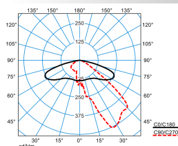
Publisca P2-AB2L/3500-740 4G1S TX047721 DIN 5040: A30 UTE: 1,00 G DLOR: 100 % ULOR: 0 % CEN Flux Code: 35 73 97 100 100
