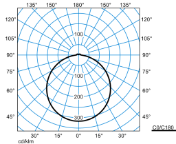
Olisq RWD4 DW 60-8TW ETDD8 IP54 + Olisq RWD4 ZDR 1/2 01 (DWW)
