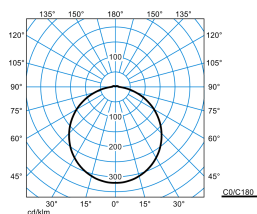
Olisq RWD4 DW 60-8TW ETDD8 IP54 + Olisq RWD4 C 01 (DCW)
