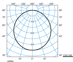
Olisq RWD4 DW 60-8TW ETDD8 IP54 + Olisq RWD4 ZDR 1/1 05 (DSU)
