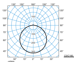
Olisq RWD4 DW 60-8TW ETDD8 IP54 + Olisq RWD4 ZDR 1/2 01 (DCW)
