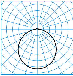
Olisq RWD4 DW 60-8TW ETDD8 IP54 + Olisq RWD4 ZDR 1/2 03 (DWW) TX874276
