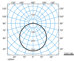
Olisq RWD4 DW 60-8TW ETDD8 IP54 + Olisq RWD4 ZDR 1/2 03 (DWW)
