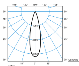
Altigo G2 60 RM3L/2000-830 1G1P + VE IP66 24V DC 60W
