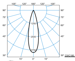
Altigo G2 60 RM3L/2000-830 1G1P + VE IP66 24V DC 80W
