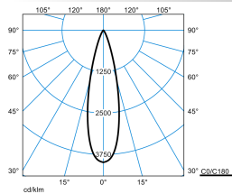
Altigo G2 60 RM3L/2000-830 1G1P + VE IP66 24V DC 250W
