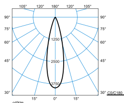
Altigo G2 60 RM3L/2000-830 1G1P + VE IP66 24V DC 130W
