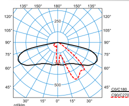
Publisca P2-AB2L-LRA/1350-740 2G1S
