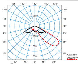
LnPlus 60-AM19L-SLR1/20000-740 16G1 ET (CLO end value) TX377652
