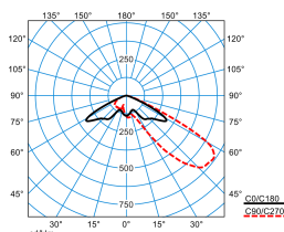
LnPlus 60-AM19L-SLR1/20000-740 16G1 ET (CLO initial value) TX376973
