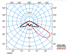
LnPlus 40-AM19L-SLR1/5100-730 6G1 ET (CLO initial value)
