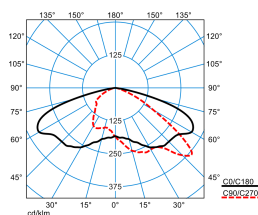
LnPlus 40-AB7L/2200-740 2G1 ETDD (CLO end value)
