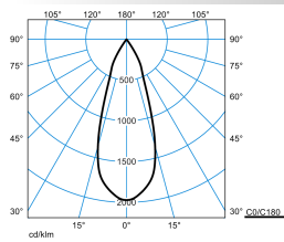
CPL G2 3P FL 30-EW M48 ET L1,5 01
