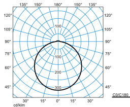
Olisq RWD4 DW 40-830 ET HFS PC + Olisq RWD4 ZDR 1/2 01
