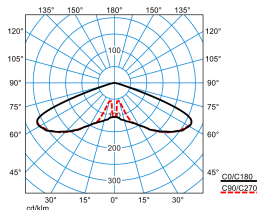
Publisca P2-RB6L-LR/1100-730 2G1S TX047844
