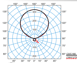
Luceos S-T PAW-IL 300-840 ETDI 05+LLWP (LEO1)
