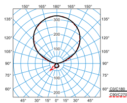
Luceos S-T PAW-IL 300-840 ETDI 05+LLWP (LEO2)
