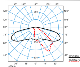
Publisca P3-AB2L-MLLR/16-42-740 4G1 ETDD (CLO initial value)
