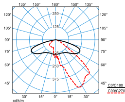
Publisca P2-AB2L/3200-730 4G1S TX047718 DIN 5040: A30 UTE: 1,00 G DLOR: 100 % ULOR: 0 % CEN Flux Code: 35 73 97 100 100
