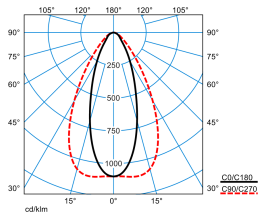
7651IP MironaF T 270-840ETDD L225 01ESG (LEO2) TX306235
