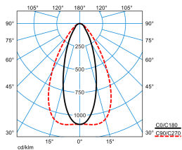
7651IP MironaF T 270-840ETDD L225 01ESG (LEO3) TX306266
