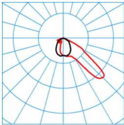
Jovie 50-AM2L-6-51-730-CLO-E
