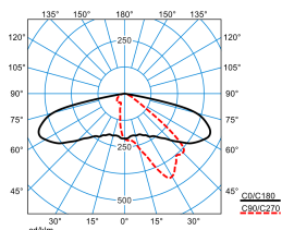
Publisca P3-AB2L-LR/6800-740 6G1 ET (CLO end value)
