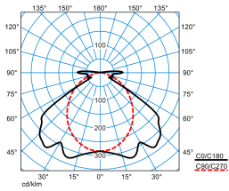
Nextrema G3 B 6000-840 ETDD +HFSB LV PC
