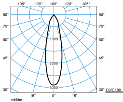
E-Line PRO 78 BV G2 RF-MF 30-BC M49 ETDD 03 Blank TX715484
