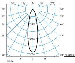
E-Line PRO 78 BV G2 RF-MF 30-BC M49 ETDD 03 03 TX715483
