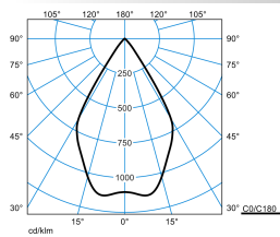
Inveria C 150 RB20R/2300-840 1G1P ETDD
