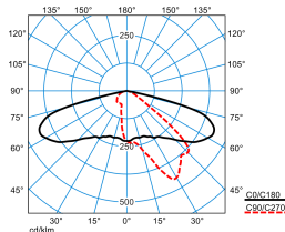
Jovie 70-AB2L24S1-120-7TW-ET-CAB-26 (DCW-CLO end value)
