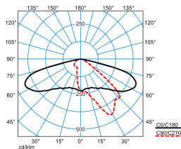
Jovie 70-AB2L24S1-120-7TW-ET-CAB-26 (DSU-CLO end value)
