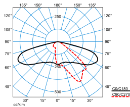
Jovie 70-AB2L24S1-120-7TW-ET-CAB-26 (DCW-CLO initial value)
