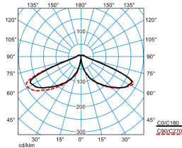
8841LS-UE 260-RB6L/1500-730 3G2 ET (CLO initial value)
