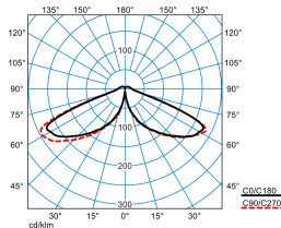
8841LS-UE 260-RB6L/1500-730 3G2 ET (CLO end value)
