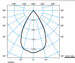
E-Line PRO 78 BV G2 RF-VFL 40-EC M39 ETDD 03
