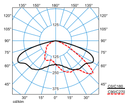
LnPlus 40-AB7L-SLR3/8200-722 8G1 ET (CLO end value)
