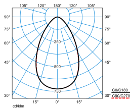
E-Line PRO 78IP50 MironaF TB 130-840 ET L150 01 01 IP50 (LEO2)
