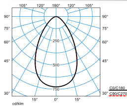
E-Line PRO 78IP50 MironaF TB 130-840 ET L150 01 01 (LEO1)
