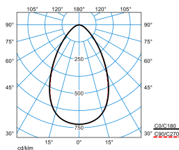
E-Line PRO 78IP50 MironaF TB 130-840 ET L150 01 01 IP50 (LEO1)
