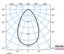
E-Line PRO 78IP50 MironaF TB 130-840 ET L150 01 01 (LEO2)
