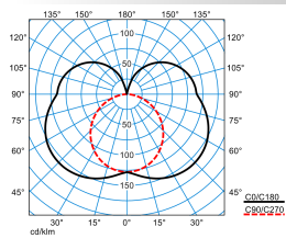
Acuro St LED1000ww ET 01 TX773684
