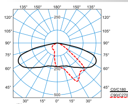
Jovie 50-AB2L-ML-LR/4600-6800-730 6G1 ET (CLO initial value)
