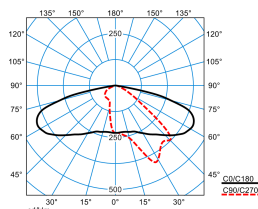
Jovie 50-AB2L-ML-LR/4600-6800-730 6G1 ET (CLO end value)
