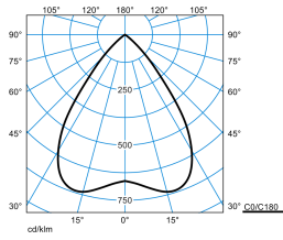
InperiaL G2 C07 BR19 2700-840 ET 01 TX768299
