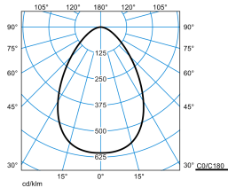
InperiaL G2 C07 BR19 2700-840 01 + DA-M 01 TX052847
