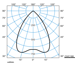
InperiaL G2 C07 BR19 2700-840 01 + DA 01 TX052846
