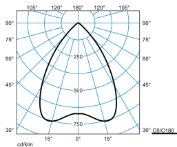
InperiaL G2 C07 BR19 2700-840 01 + RD-PC TX052848
