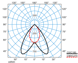
Creavo M314-TS CLDAW-01 80-830 ET 01
