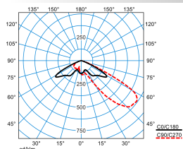
LnPlus 40-AM19L-SLR1/10000-727 8G1 ET (CLO end value) TX376832
