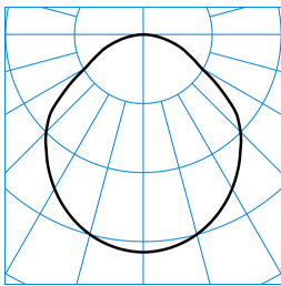
Inplana C07 OTA22 1000-830 ETDD 01 ■ C0 - C180 TX772407
