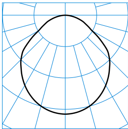
Inplana C07 OTA22 1000-830 01 + C07 ZPF - T ■ C0 - C180 TX772405
