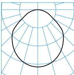
Inplana C07 OTA22 1000-830 01 + C07 ZPF - T WR ■ C0 - C180 TX772406
