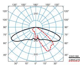
Publisca P2-AB2L/5100-730 6G1S ETDD (CLO end value)
