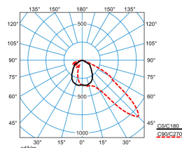
Jovie 50-AM2L-4-42-730-CLO-E
