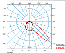
Jovie 50-AM2L-4-42-730-CLO-B
