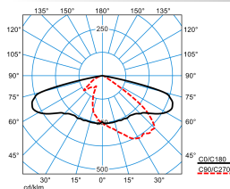
LIQ 70N-AB7L-LR/7500-722 8G1 ET (CLO end value) TX778331
