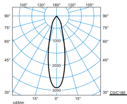
E-Line PRO 78 BV G2 RF-MF 20-M M52 ETBLE 03 Blank
