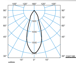
E-Line PRO 78 BV G2 RF-FL 20-BC M49 ET 05 05
