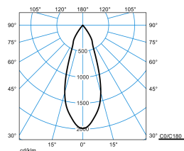
E-Line PRO 78 BV G2 RF-FL 20-BC M49 ET 05 Blank
