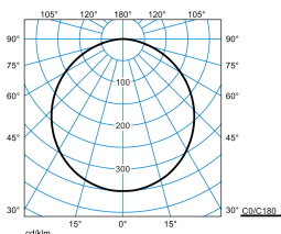
Olisq RWD3 DW 30-840 ETDD PC + Olisq RWD3 ZVF 01
