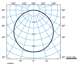
Olisq RWD3 DW 30-840 ETDD PC + Olisq RWD3 ZDR 1/1 01
