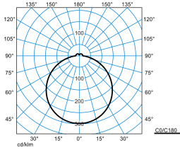
Olisq RWD3 DW 30-840 ETDD PC
