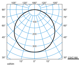
Olisq RWD3 DW 30-840 ETDD PC + Olisq RWD3 ZDR 1/1 05
