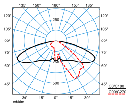
Publisca P2-AB2L-LR/5100-730 6G1S ET (CLO end value) TX300348 DIN 5040: A30 UTE: 1,00 G DLOR: 100 % ULOR: 0 % CEN Flux Code: 35 74 97 100 100
