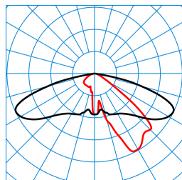
Publisca P2-AB2L-LR/5100-730 6G1S TX047765 ■ C0 - C180 ■ C90 - C270 DIN 5040: A30 UTE: 1,00 G DLOR: 100 % ULOR: 0 % CEN Flux Code: 35 74 97 100 100
