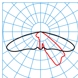
Publisca P2-AB2L-LR/5100-730 6G1S ET (CLO end value) TX300348 ■ C0 - C180 ■ C90 - C270 DIN 5040: A30 UTE: 1,00 G DLOR: 100 % ULOR: 0 % CEN Flux Code: 35 74 97 100 100
