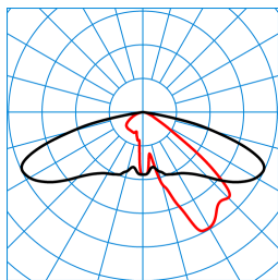
Publisca P2-AB2L/5100-730 6G1S ETDD (CLO initial value) TX300337 ■ C0 - C180 ■ C90 - C270 DIN 5040: A30 UTE: 1,00 G DLOR: 100 % ULOR: 0 % CEN Flux Code: 35 74 97 100 100
