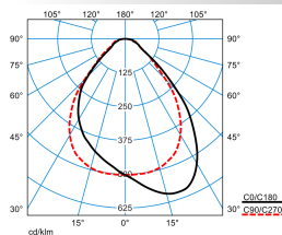
ArimoFit G2 D2 P-WW 42-840 ET 03/03
