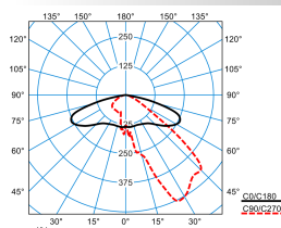
Publisca P1-AB2L/2900-730 4G1S
