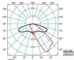
Publisca P1-AB2L/2900-730 4G1S ETDD (CLO end value)
