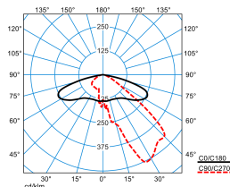
Publisca P1-AB2L/2900-730 4G1S ETDD (CLO end value)
