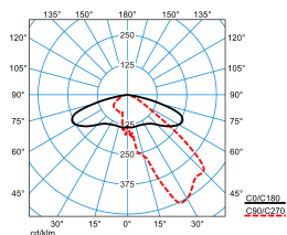
Publisca P1-AB2L/2900-730 4G1S
