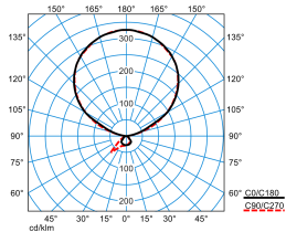
Luceos S-T PAW-IL 300-840 ETDD 03 (LEO2) TX877123
