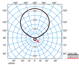
Luceos S-T PAW-IL 300-840 ETDD 03 (LEO1) TX877112
