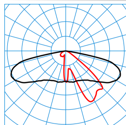
Publisca P2-AB2L/1350-740 2G1S TX047701 ■ C0 - C180 ■ C90 - C270 DIN 5040: A30 UTE: 1,00 G DLOR: 100 % ULOR: 0 % CEN Flux Code: 34 70 96 100 100
