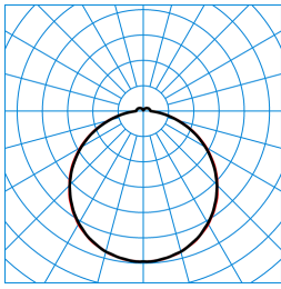
Olisq QWD2 DW 14-40/4/ML-830 IP54 ET + Olisq QWD2 ZDR 1/2 01 (stage 1) TX462164
