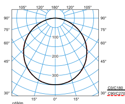
Olisq QWD2 DW 14-40/4/ML-830 IP54 ET + Olisq QWD2 ZDR 1/1 01 (stage 3)
