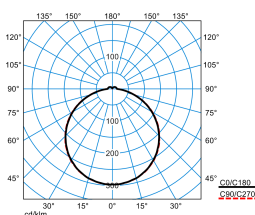
Olisq QWD2 DW 14-40/4/ML-830 IP54 ET + Olisq QWD2 ZDR 1/2 03 (stage 3)
