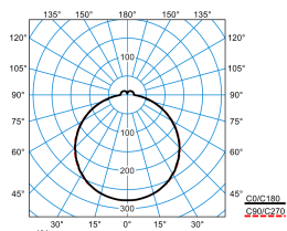
Olisq QWD2 DW 14-40/4/ML-830 IP54 ET (stage 3)
