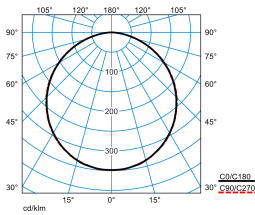
Olisq QWD2 DW 14-40/4/ML-830 IP54 ET + Olisq QWD2 ZDR 1/1 03 (stage 1)
