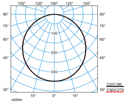
Olisq QWD2 DW 14-40/4/ML-830 IP54 ET + Olisq QWD2 ZDR 1/1 01 (stage 1)
