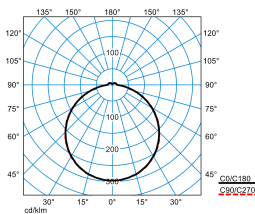
Olisq QWD2 DW 14-40/4/ML-830 IP54 ET + Olisq QWD2 ZDR 1/2 01 (stage 3)
