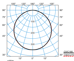
Olisq QWD2 DW 14-40/4/ML-830 IP54 ET + Olisq QWD2 ZDR 1/1 03 (stage 3)
