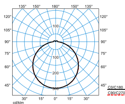
Olisq QWD2 DW 14-40/4/ML-830 IP54 ET + Olisq QWD2 ZDR 1/2 03 (stage 3)
