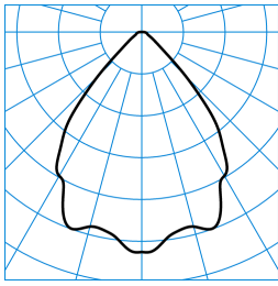
InperiaLP C05 HR22 1800-840 01 + ZN-PC ■ C0 - C180 TX041704
