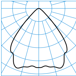
InperiaLP C05 HR22 1800-840 01 + RG-PC TX041703
